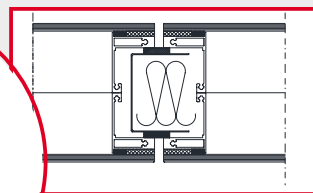
Detailschnitt Glasrahmen Planus clear
